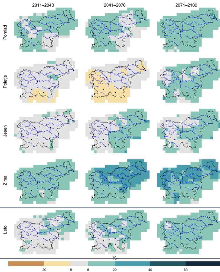
RCP4.5
