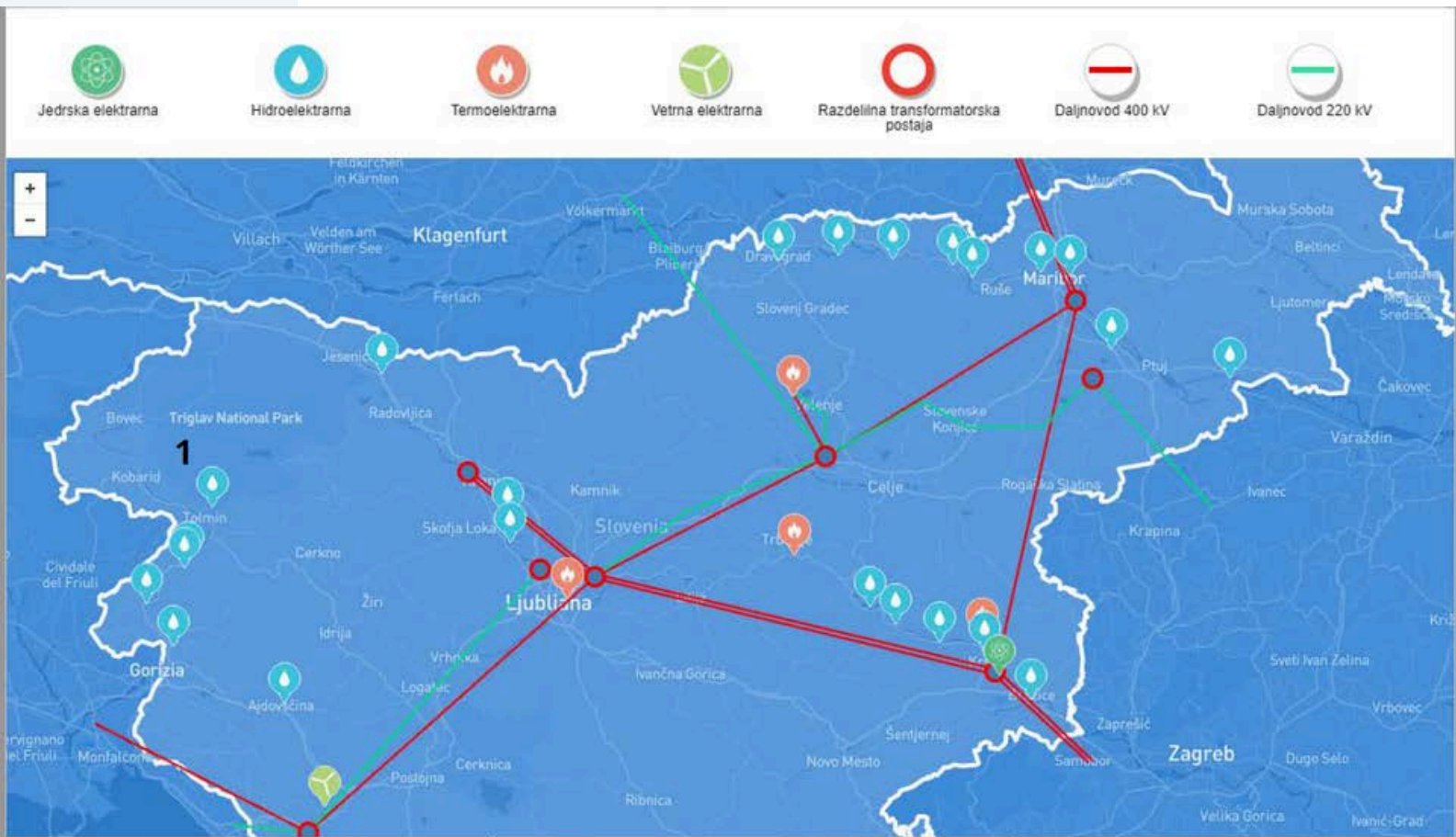
Slika: Elektroenergetski sistem Slovenije; Vir: esvet.si
