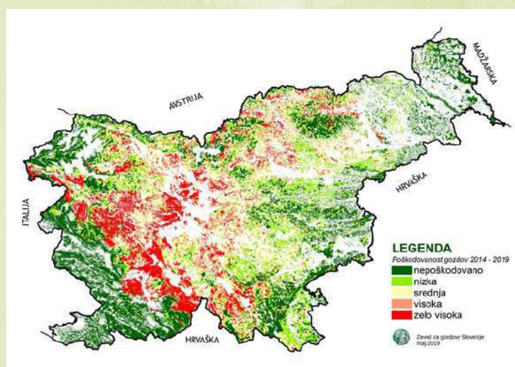
Slika 23: Poškodovanost gozdov 2014-2019
